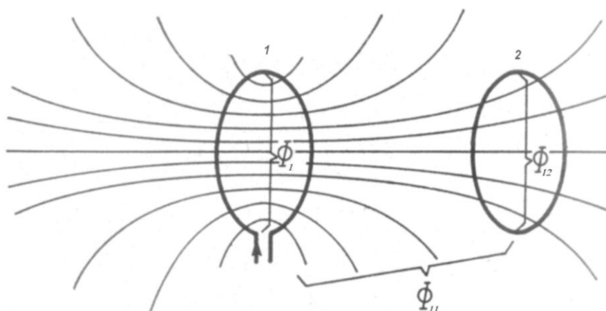
Rys. 1. Strumień magnetyczny \Phi_1 wytwarzany przez cewkę i jego podział na \Phi_{12} i \Phi_{11}
